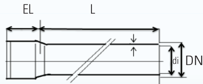
Rigid Electrical Conduit
